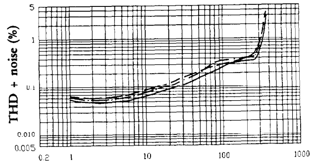
Output (Watts)
